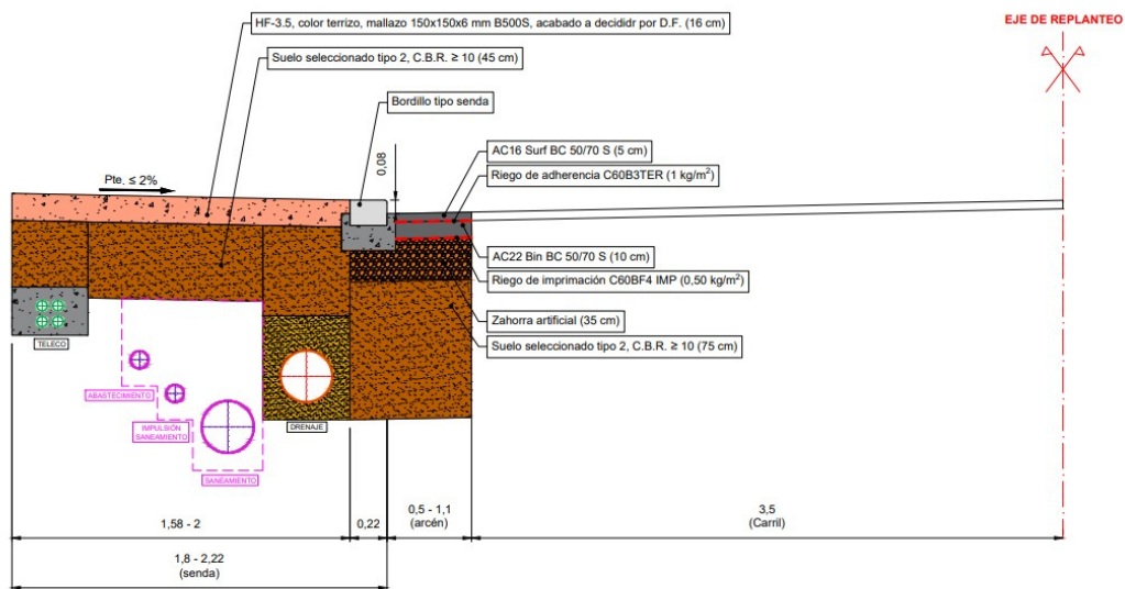
Sección tipo senda
